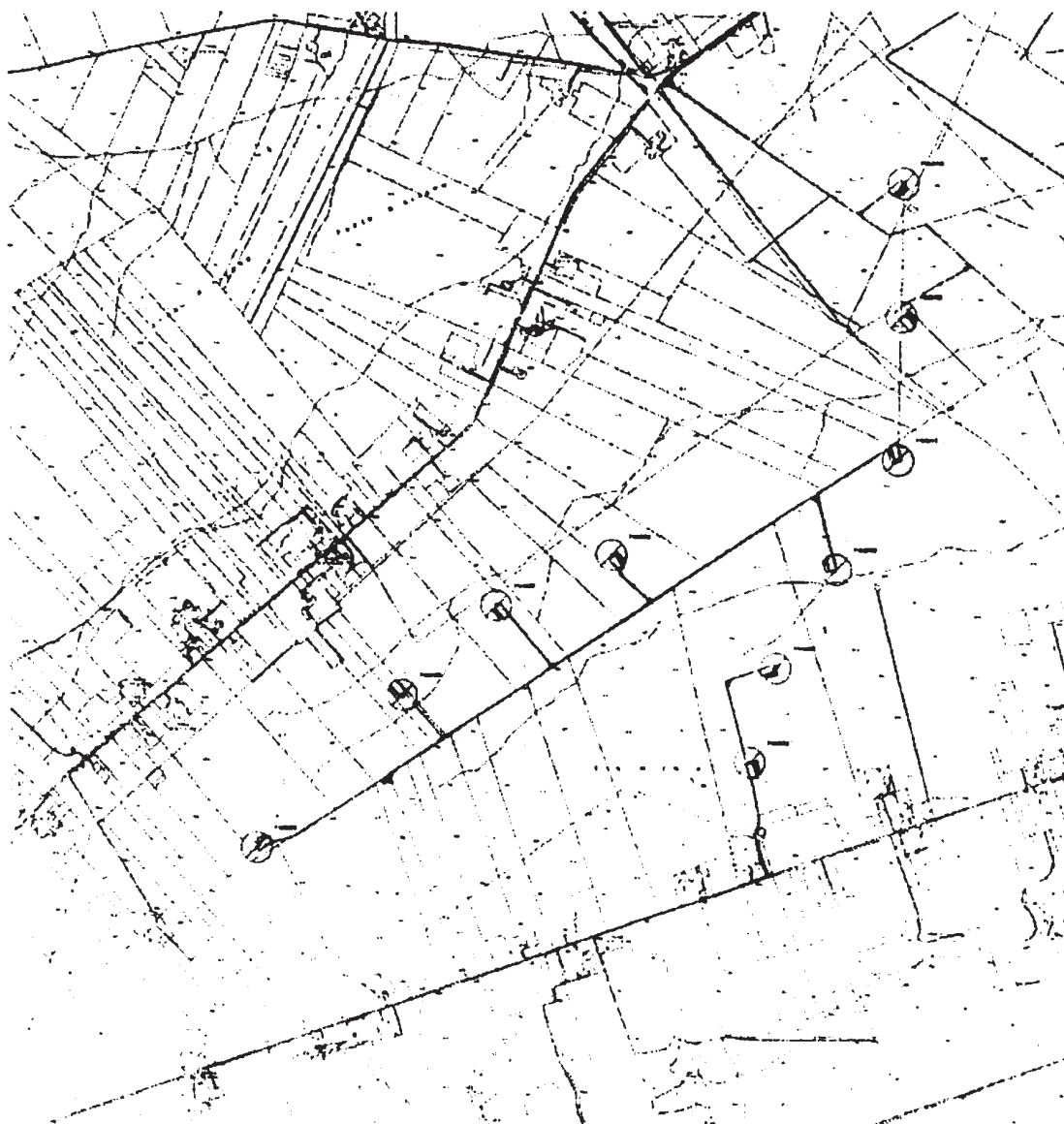
Figura 2 Inquadramento su CTR – Layout da 10 aerogeneratori
